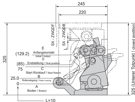
Ansicht mit Treiber View with driver
