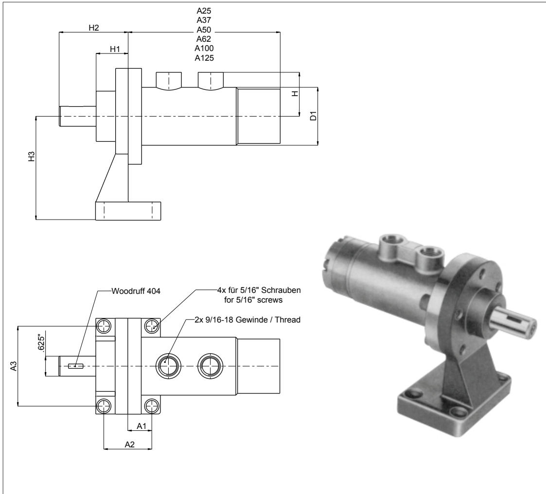
Abmessungen / Dimensions
