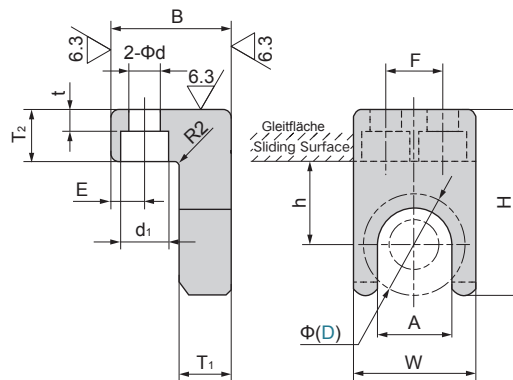
⑤ Rückführungsplatte Return Plate
